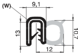
PA7400057-000 **mm. 1,5 a 2,5 SILICONE COMPACT + SPONGE + METAL
