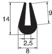
PA7100770-000 EPDM
