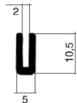
PA7200361-000 PVC
