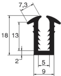
PA7100774-000 EPDM
