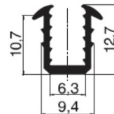
PA7101422-000 EPDM
