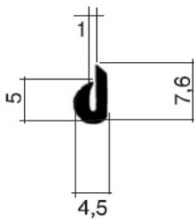
PA7200046-000 PVC
