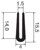
PA7100620-000 EPDM
