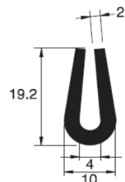
PA7100631-000 EPDM
