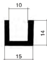
PA7100556-000 EPDM
