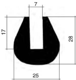
PA7100913-000 EPDM
