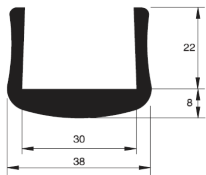
PA7100779-000 EPDM
