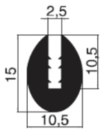
PA7200176-000 PVC
