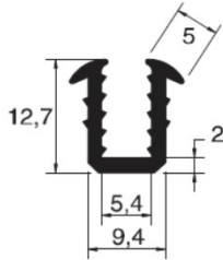
PA7100757-000 EPDM
