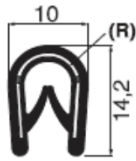
PA7200480-000 **mm. 1 a 4 PVC
