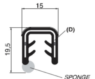
PA7101191-000 **mm. 4 a 7 EPDM
