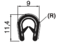
PA7200530-000 **mm. 2 a 4 PVC
