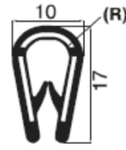
PA7200294-000 PA7200281-000 **mm. 1 a 4 PVC
