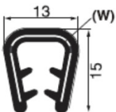
PA7102036-000 **mm. 5 a 6 EPDM
