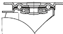
Rolamento na coroa giratória:
