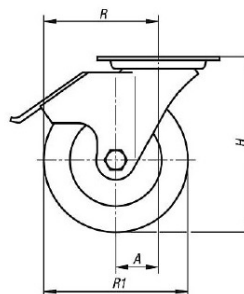
Rodízio giratório com freio "stop-fix"
