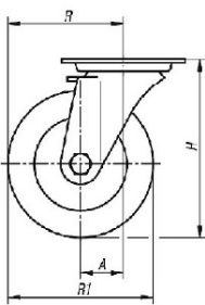
Rodízio industrial giratório
